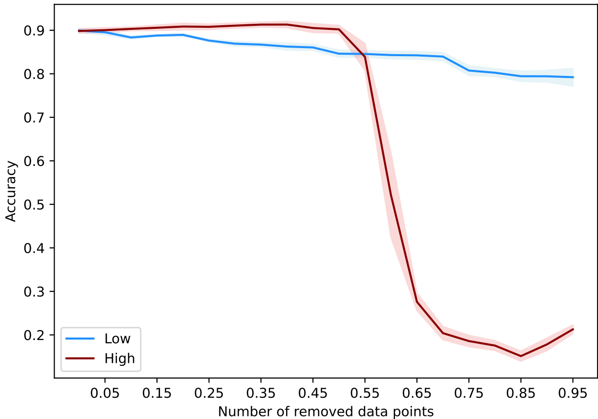
DataOob(1000, epochs=15) - nomao
